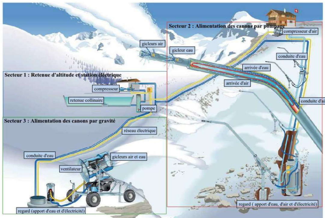
Schéma de l'installation d'un réseau d'enneigement (P. Paccard, 2010)
