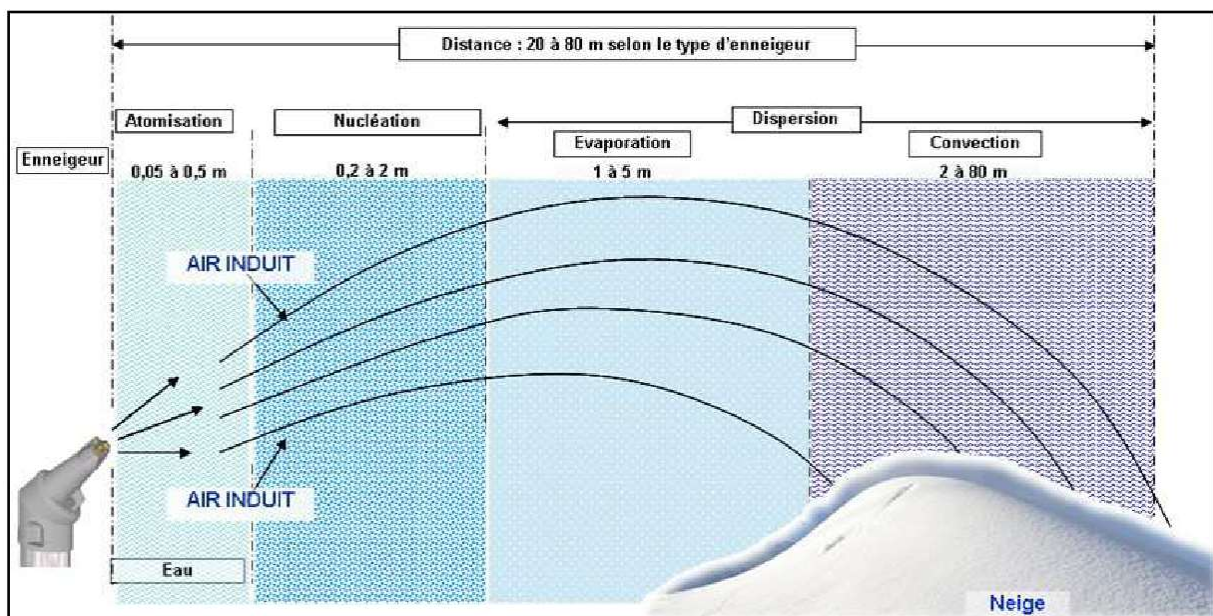
Schéma des différentes phases de production de neige (SNTF, 2002)
